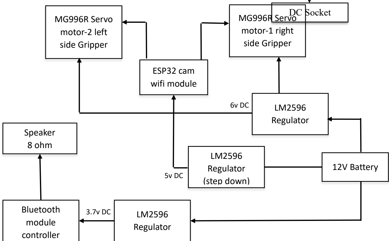
Fig: a) Bottom circuit
